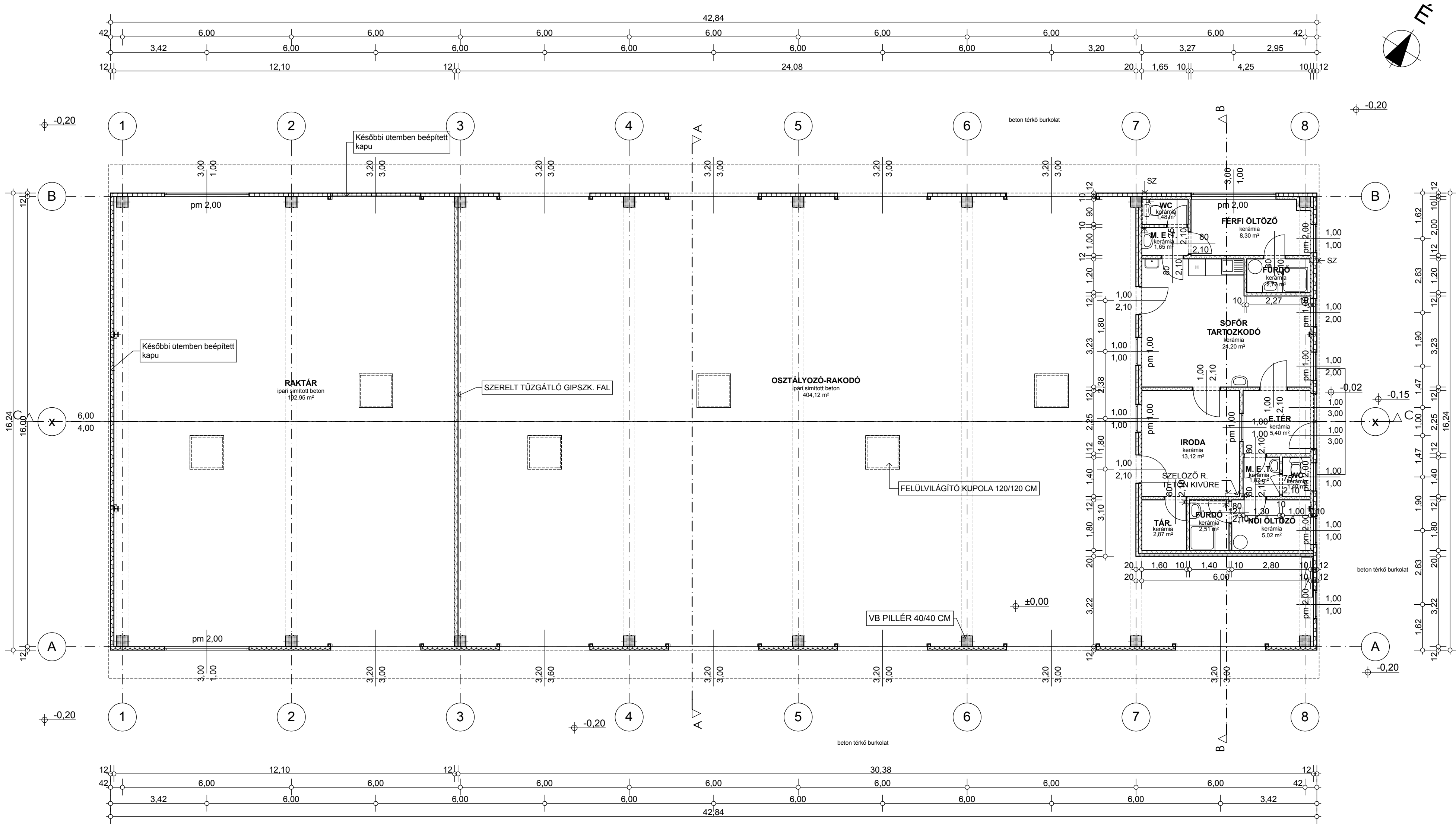
FÖLDSZINTI ALAPRAJZ M=1:100
